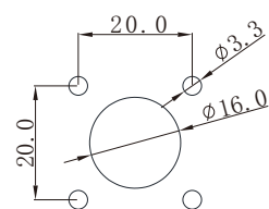
开孔尺寸
